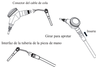
Figura 4 Conexión del cable de cola
