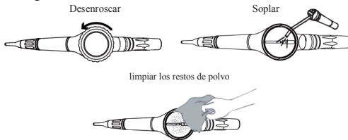
Figura 9 Diagrama esquemático de la limpieza del polvo
