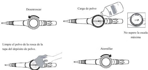
Figura 6 Carga de polvo
